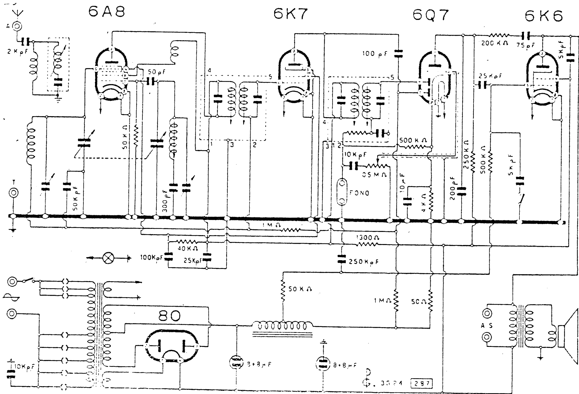
UNDA RADIO - MOD. « MONO UNDA 511 »
